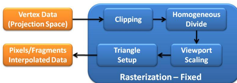
Figura3: Estágio de rasterização.
