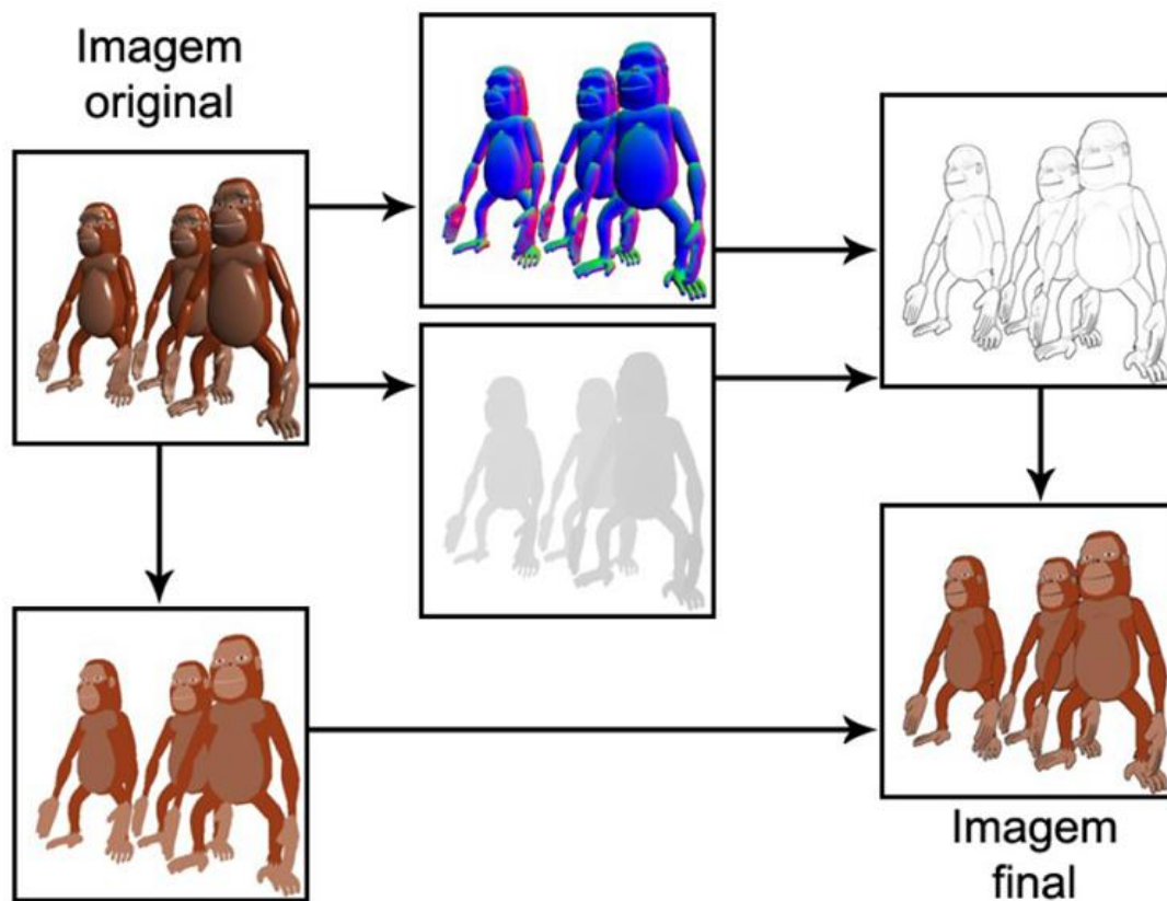
Figura 34: Diagrama do processo de cartoon rendering.
