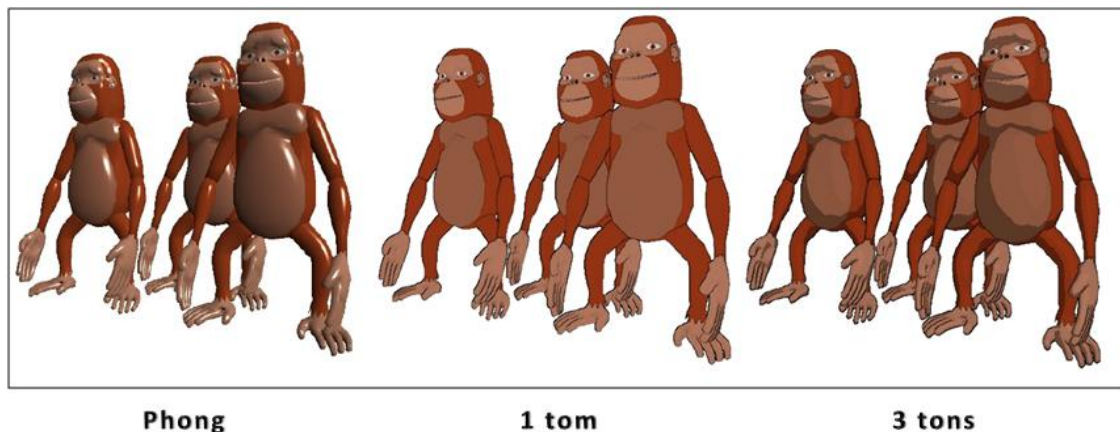
Figura 32: Exemplo de renderização de cartoon com aplicação de quantização de 1 tom e de 3 tons .
