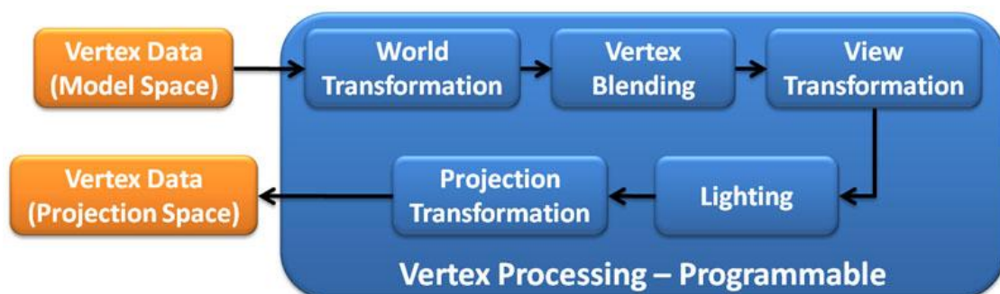
Figura 2: Estágio de processamento de vértices.
