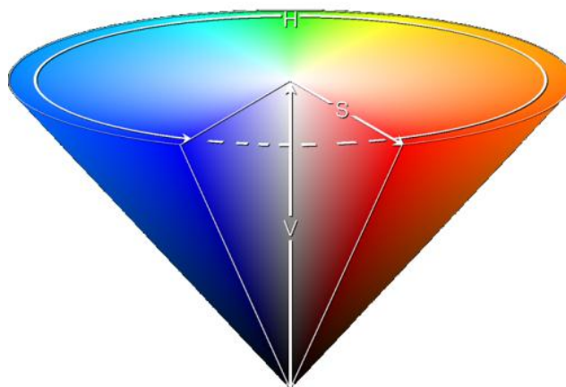
Figura 24: Representação do espaço de cor HSV em formato de cone.
