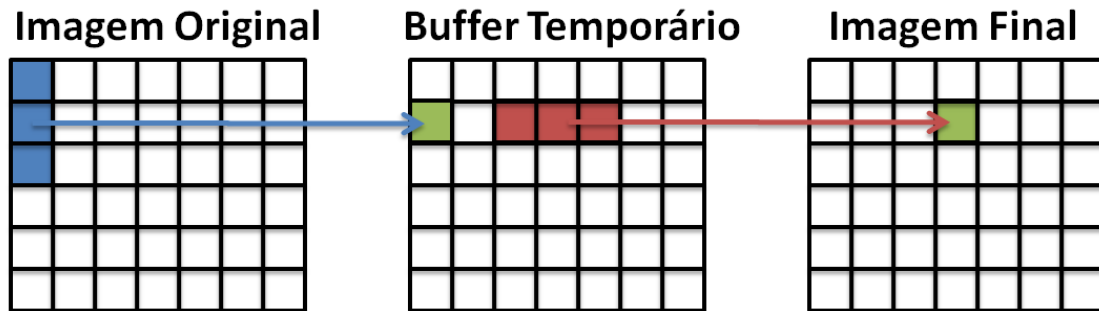
Figura 29: Diagrama do algoritmo otimizado de blur
