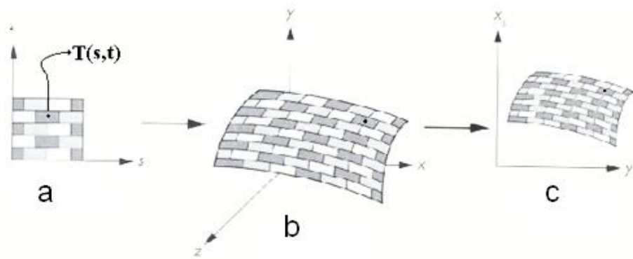
Figura 9: Mapeamento de textura. a) função textura 'T' que recebe as coordenadas 's' e 't' e endereçam uma determinada cor; b) objeto3D que possui um dado mapeamento para o espaço de 'T'; c) imagem final que utiliza os texels de 'a' para atribuir cor aos pixels.
