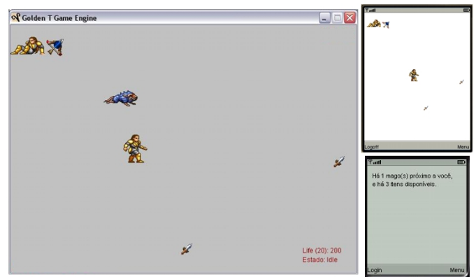
Figura 10: Diferentes visões de um estado do jogo, de acordo com o dispositivo do jogador
