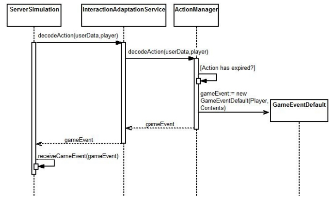
Figura 8: Diagrama de seqüência - Enviar ação de um jogador pelo Serviço de Adaptação de Interação
