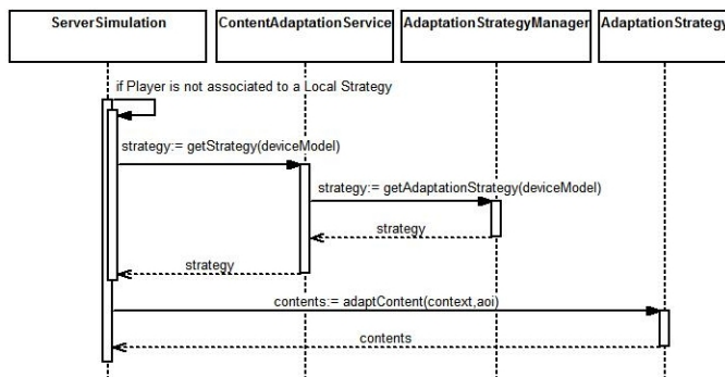
Figura 4: Diagrama de sequência da operação getStrategy do Serviço de Adaptação de Conteúdo
