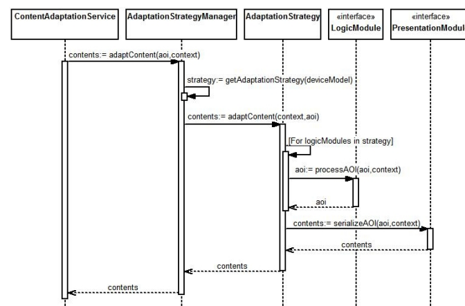
Figura 3: Diagrama de seqüência do Serviço de Adaptação de Conteúdo
